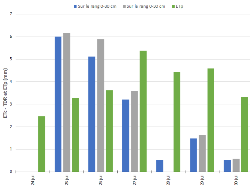
Figure 7. Évapotranspiration de la culture estimée par TDR ( ET_{c-TDR} ) (mm), évapotranspiration potentielle ( ET_p ), site IO, 24 au 30 juillet 2022.
