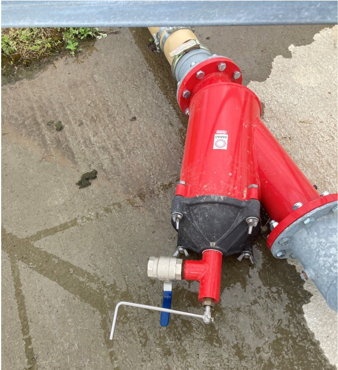
Figure 20. Filtreur Amiad installé sur la ligne d'arrivée d'eau du pivot.
