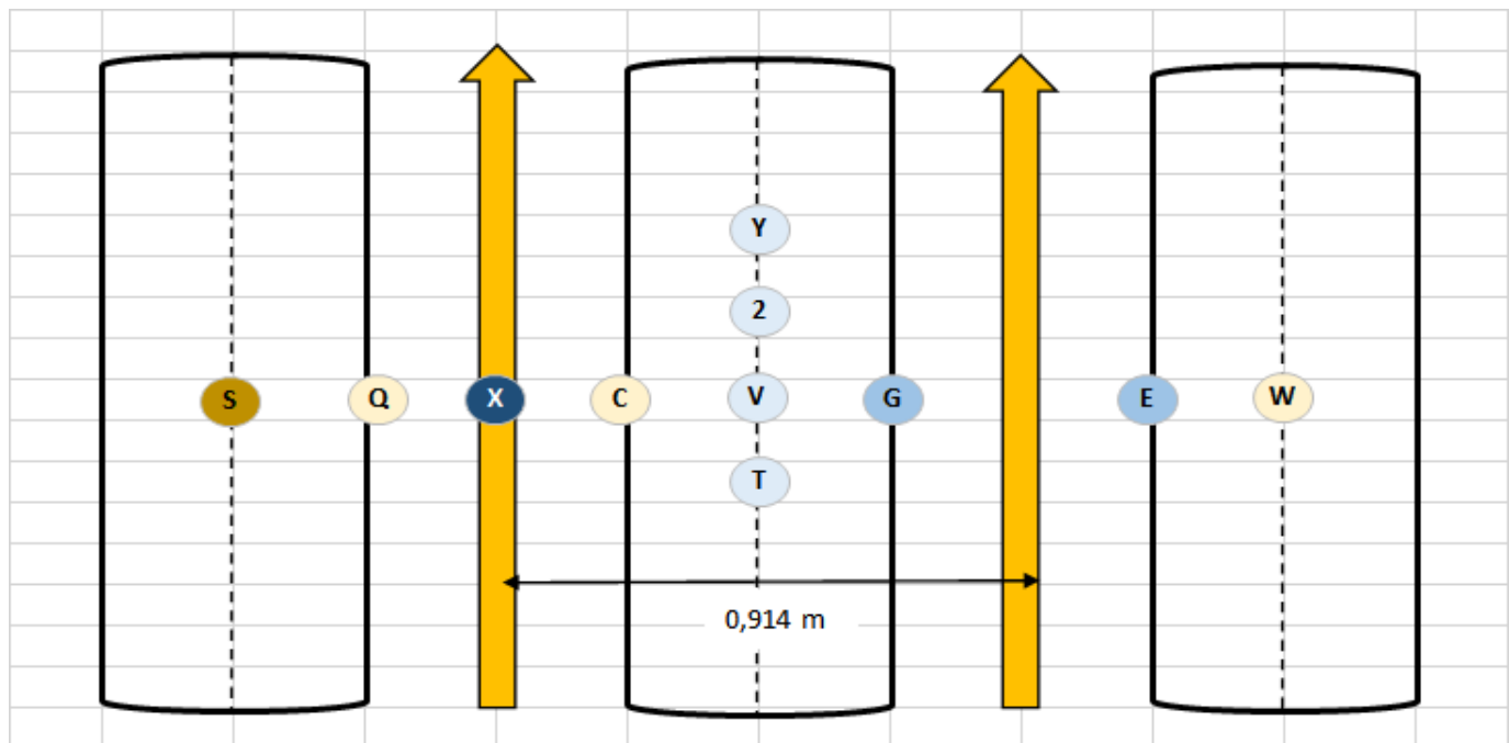
Figure 8. Disposition des 11 sondes TDR dans le système cultural en configuration « parallèle aux billons ».
